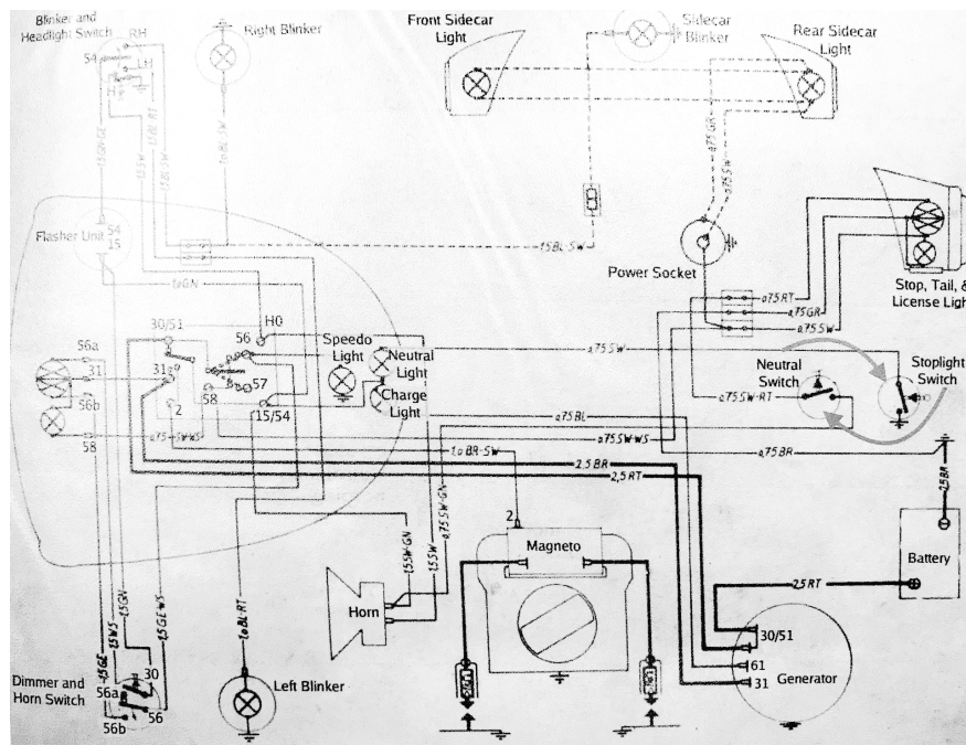
Abbildung 1 Originalschaltplan von der R69S.
