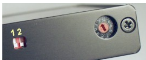
Abbildung 2 DIP-Schalter und Drehschalter.
