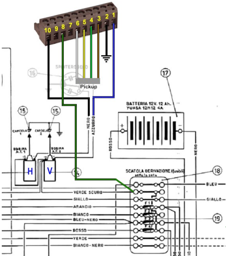
Anschluss im Stromlaufplan
