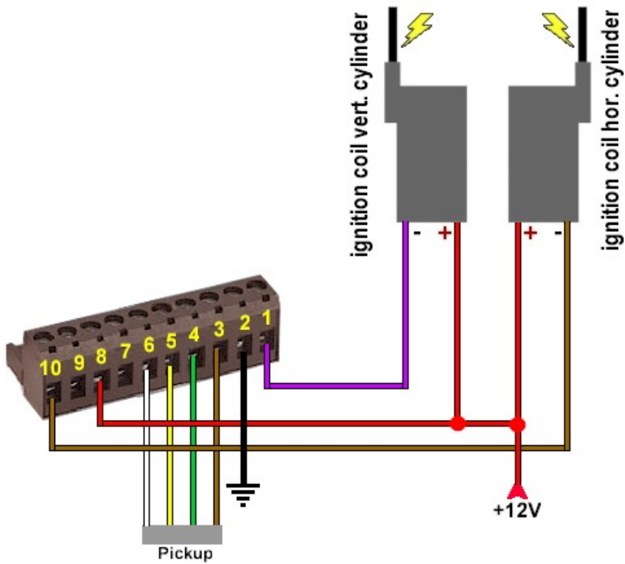
Anschlussplan
