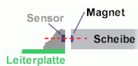
Abbildung 9 Ausrichtung von Magnetring und Sensor.
