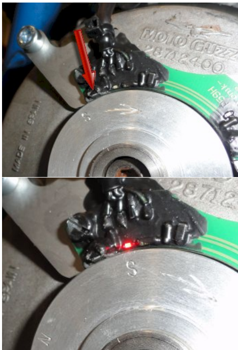
Abbildung 8 Ausrichten des Magnetringses so daß die LED gerade an- bzw. ausgeht.
